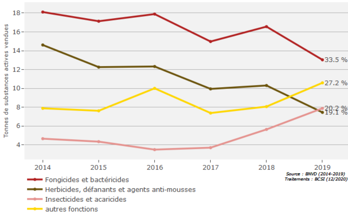
QSA par fonction de substance (en tonnes) dans les ALPES-MARITIMES
