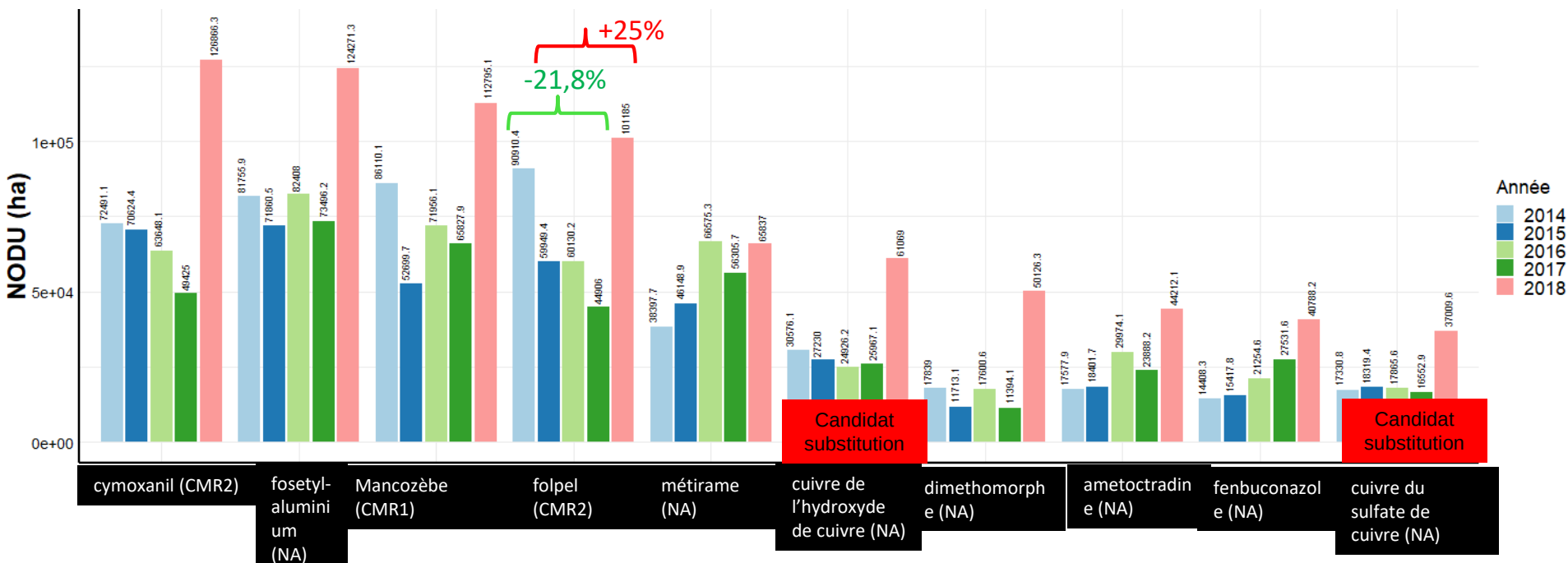
Figure 3. Evolution des NODU des substances actives les plus utilisées pour l'usage fongicide.
