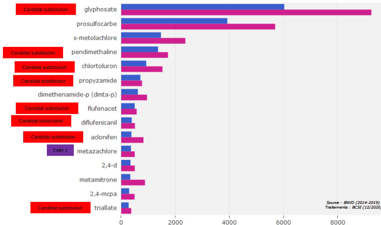
15 principales substances herbicides vendues (en tonnes) en France
