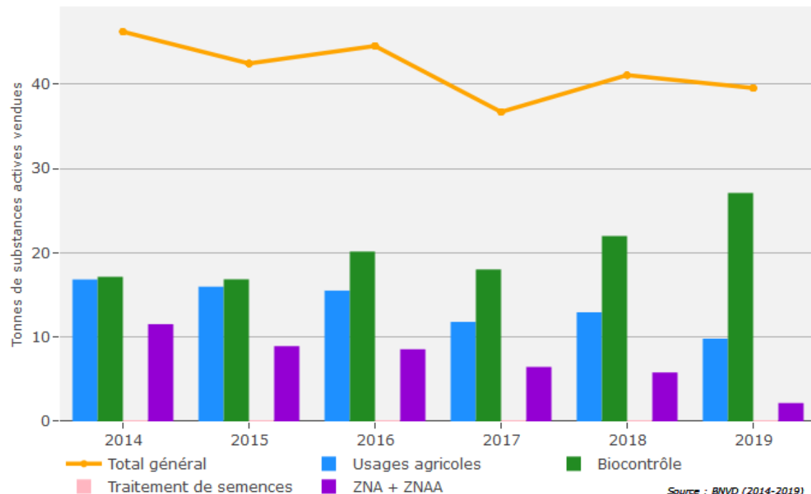
QSA totale et par segment (en tonnes) dans les ALPES-MARITIMES
