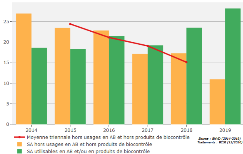
Quantité de Substances Actives vendues par type d'usages ALPES-MARITIMES (en tonnes)
