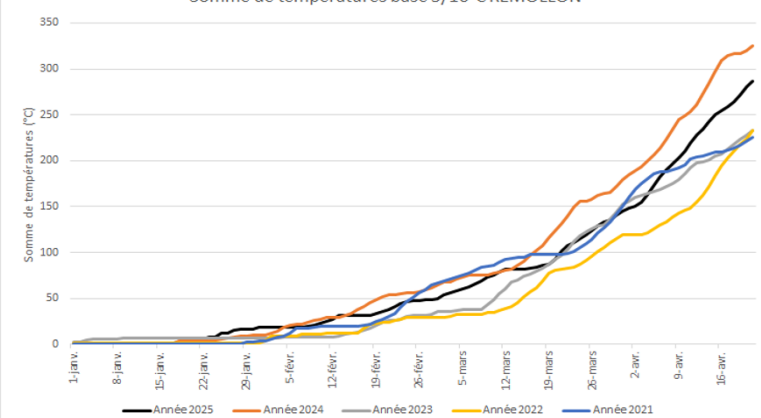
Somme de températures base 5/10°C REMOLLON
