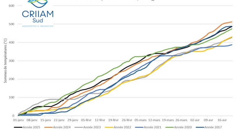
Sommes de températures base5/10°C _ BERRE
