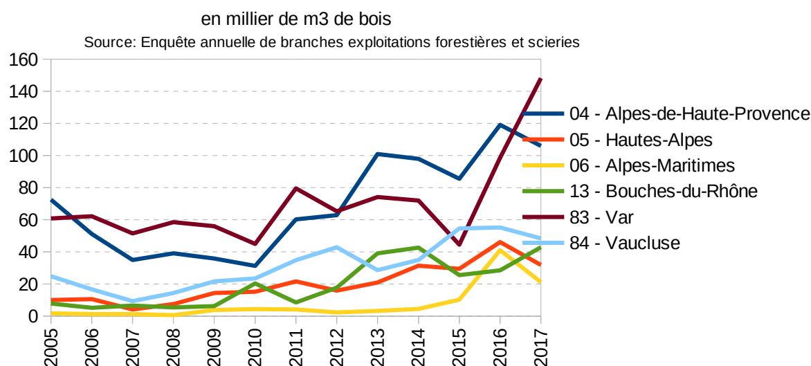
Graphique 9 : Évolution de la récolte de bois énergie par département entre 2005 et 2017
