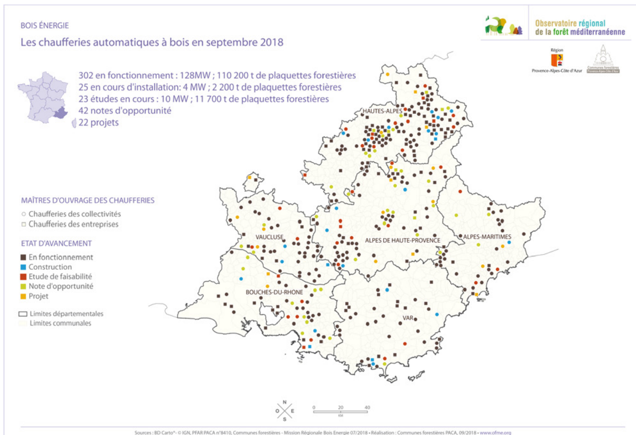
Graphique 8 : Les chaufferies-bois implantées en Provence-Alpes-Côte d'Azur en 2018
